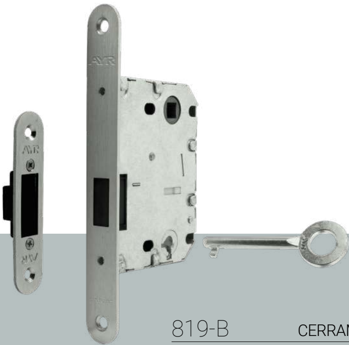
819 CERRAMAGIC Picaporte magnético unificado Níquel satinado, Latonado satinado, Negro mate, Blanco mate Entre centros 70 mm Frente/centros 50 mm
